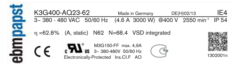
Bild 14 Typenschild des Ventilator- systems mit EC-Motor
