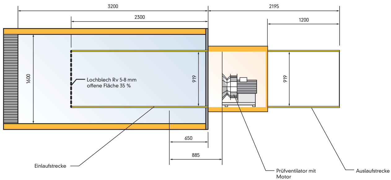
Bild 2 Darstellung der Einbaubedingungen im Kammerprüfstand
