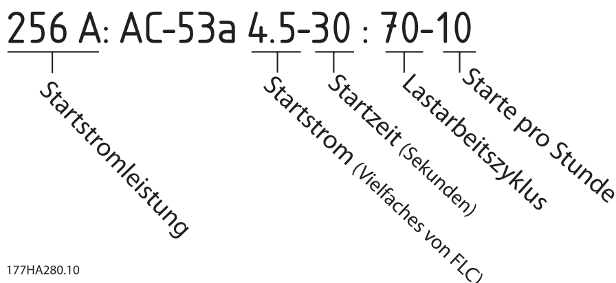
Abbildung 4.17 AC-53 Nennwerte für Dauerbetrieb
