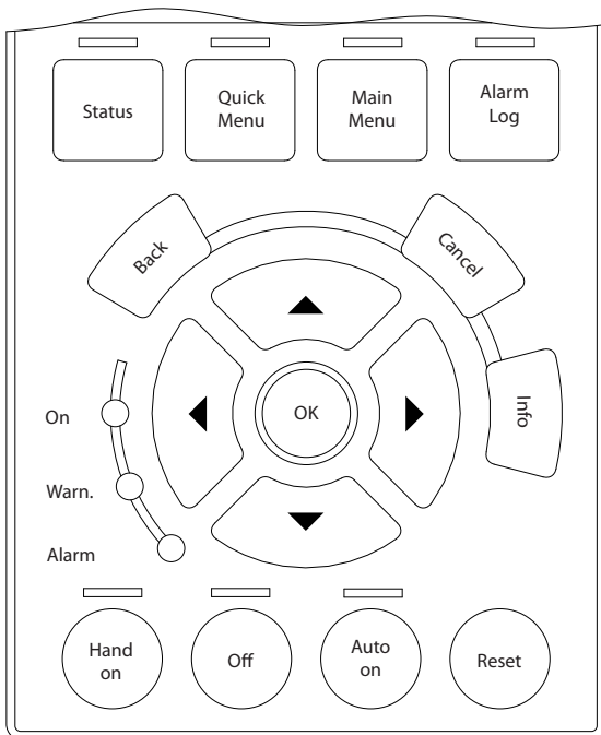
Abbildung 2.9 LCP
