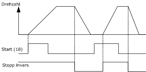
Abbildung 1.7 Puls-Start/Stopp
