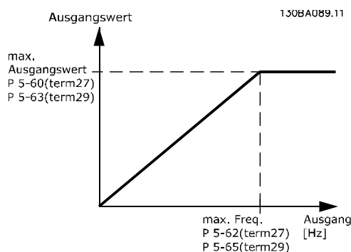
Abbildung 3.38 Konfiguration der Pulsausgänge
