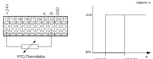
Abbildung 3.17 Thermistorverbindung
