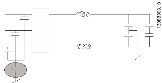
Abbildung 3.60 EMV-Filter
