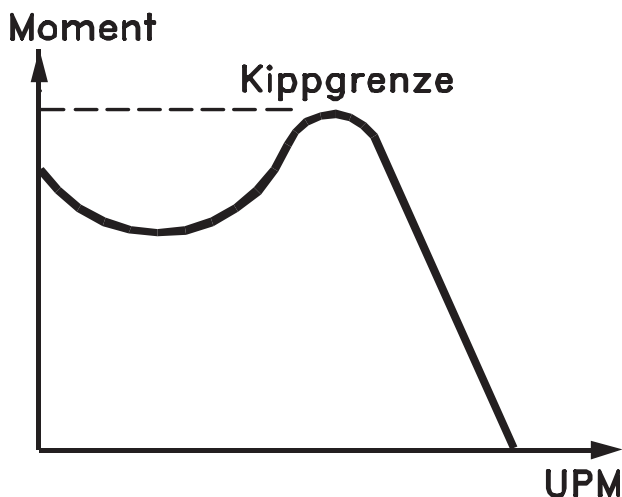
Abbildung 1.1 Losbrechmoment
