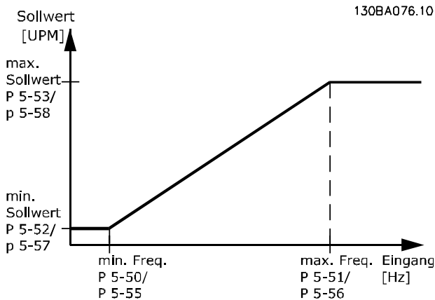
Abbildung 3.37 Pulseingänge
