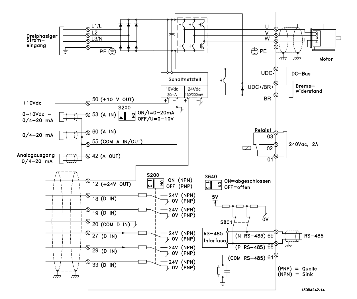
Abbildung 3.10: Elektrische Installation, Übersicht
