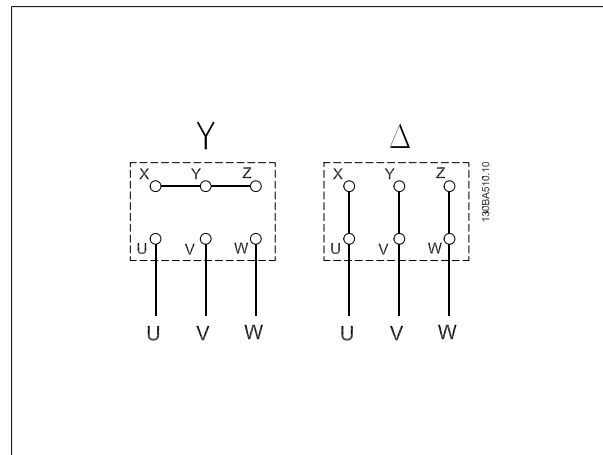
Abbildung 3.3: Stern- und Dreieckschaltung
