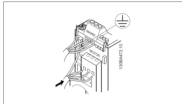
Abbildung 3.4: Befestigung von Erd- und Motorkabeln.
