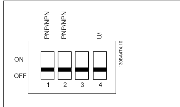
Abbildung 3.9: Schalter S200 1-4
