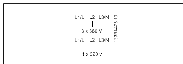
Abbildung 3.2: Kabelanschluss bei dreiphasigem und einphasigem Netzeingang.
