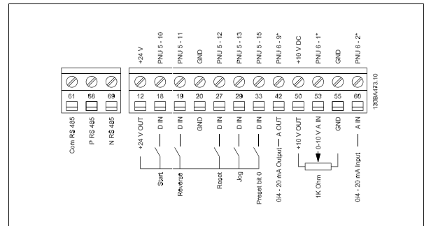
Abbildung 3.7: Übersicht von Steuerklemmen in PNP-Konfiguration und Werkseinstellung
