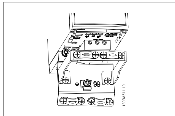
Abbildung 3.5: VLT Micro Drive mit Abschirmblech
