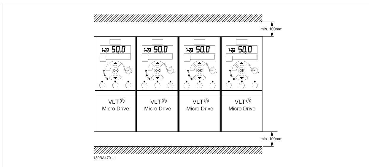
Abbildung 2.2: Einbau nebeneinander
