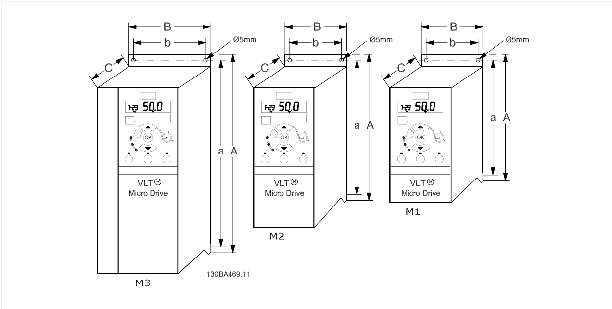
Abbildung 2.3: Abmessungen
