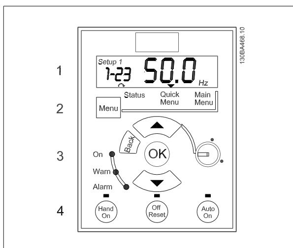
Abbildung 4.1: LCP 12 mit Potentiometer
