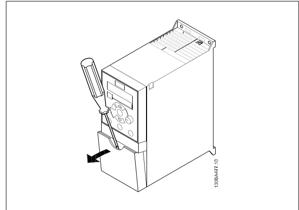
Abbildung 3.6: Entfernen der Klemmenabdeckung
