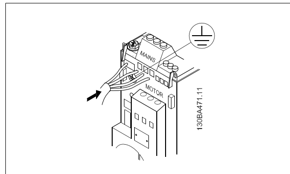
Abbildung 3.1: Netzanschluss und Erdung
