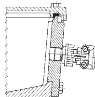
Ausführung 2 Kabeleinführungsstutzen nach EN 60079-7, mit Zugentlastung, Verdreh- und Knickschutz für das Kabel des ortsveränder- lichen Betriebsmittels
