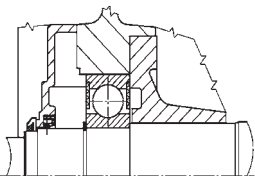
Baugröße 250
