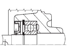
Baugröße 80–132
