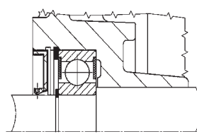
Baugröße 160
