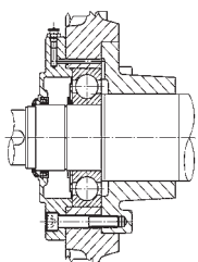
Baugröße 315–450
