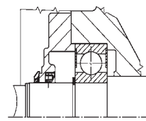
Baugröße 225
